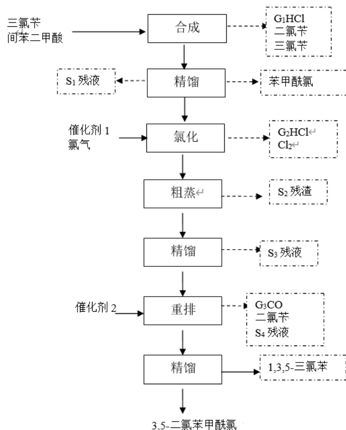
图 4.2-8 3,5-二氯苯甲酰氯联产苯甲酰氯、1,3,5-三氯苯生产工艺流程图
