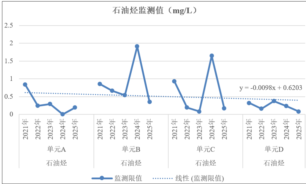
图 8.2-1 地下水监测井中石油烃监测值变化及趋势分析图
