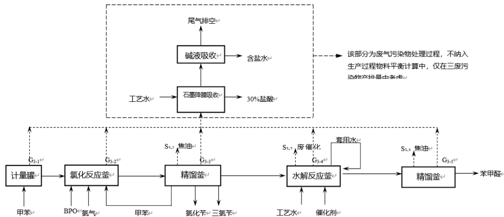
图 4.2-7 苯甲醛生产工艺流程图
