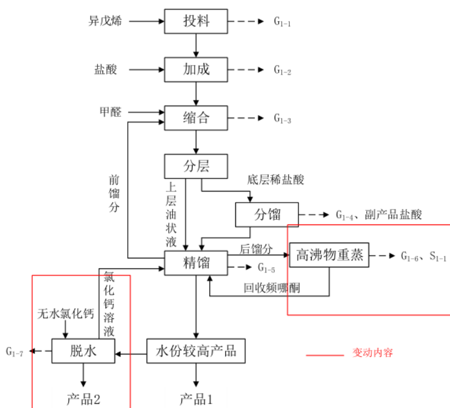
图 4.2-2 甲基叔丁基甲酮生产工艺流程图
