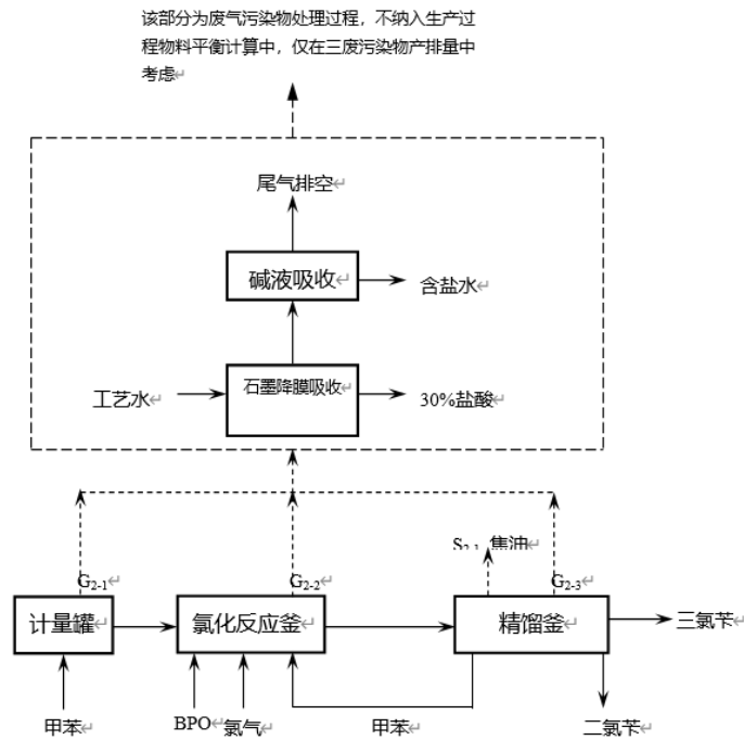
图 4.2-6 三氯苯生产工艺流程图
