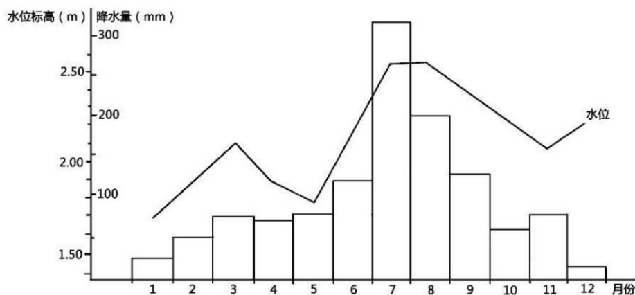
图 3.1-3 潜水位与降水量变化曲线图
