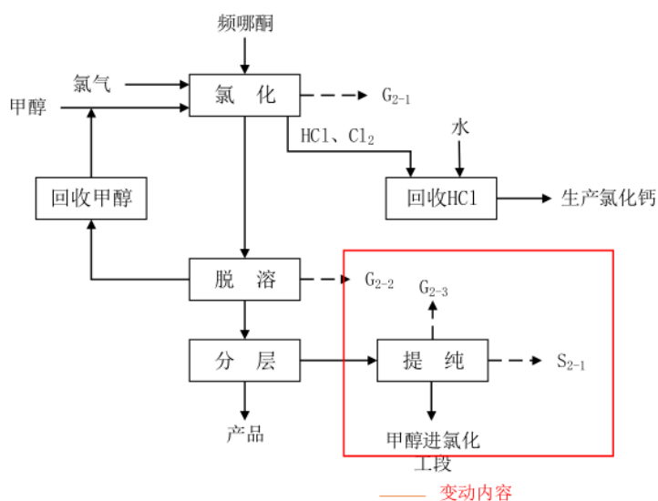
图 4.2-3 一氯频哪酮生产工艺流程图
