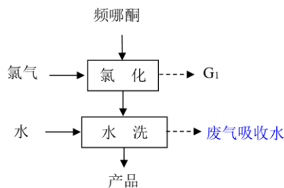
图 4.2-1 二氯频哪酮生产工艺流程图
