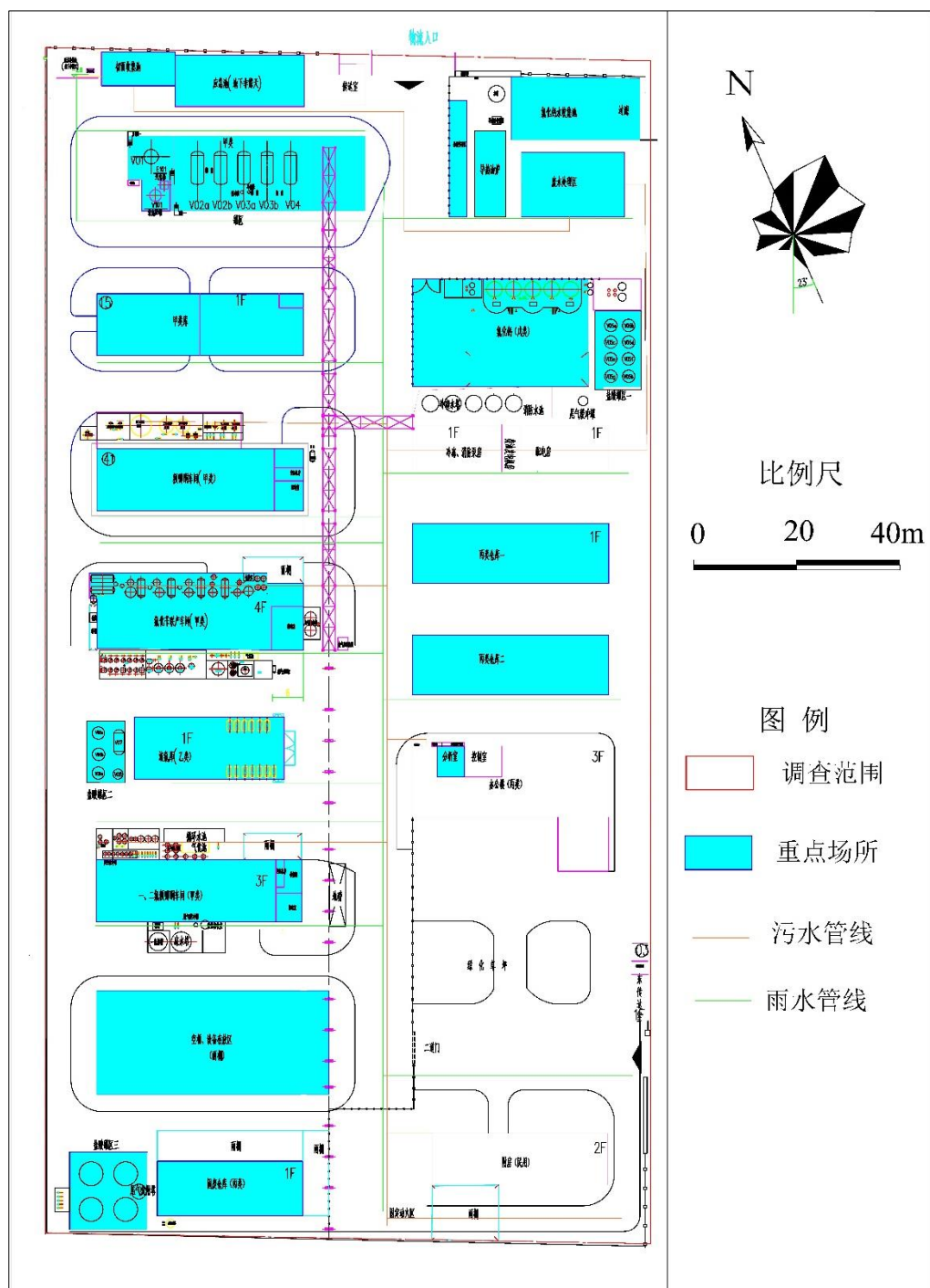
图 4.4-1 全厂总平面布置图
