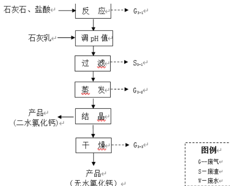
图 4.2-4 氯化钙生产工艺流程图
