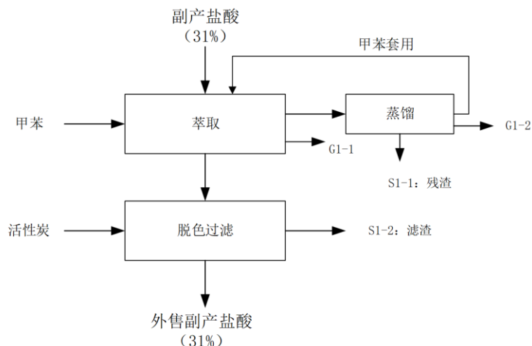
图 4.2-9 副产盐酸后处理生产工艺流程图
